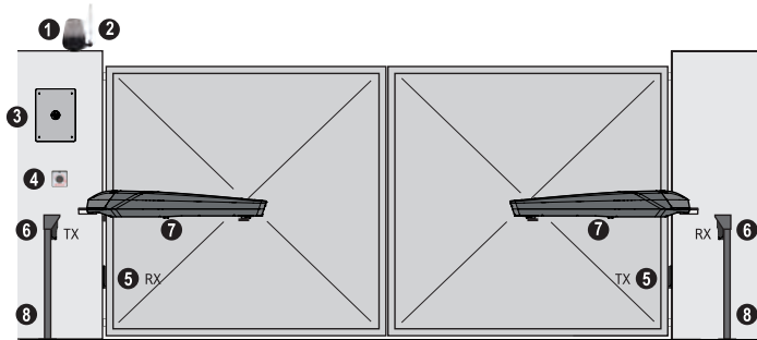
1_Lampe clignotante 2_Antenne 3_Carte de gestion 4_Contacteur à clé 5_Phocellule en FERMETURE 6_Phocellule en OUVERTURE 7_Moteurs 8_Potelet photocellule
