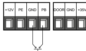
Fig. 38 - INTERRUTTORE NA
