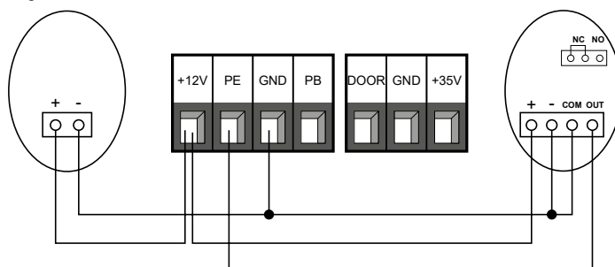
Fig. 37 - FOTOCELLULE NA/NC
